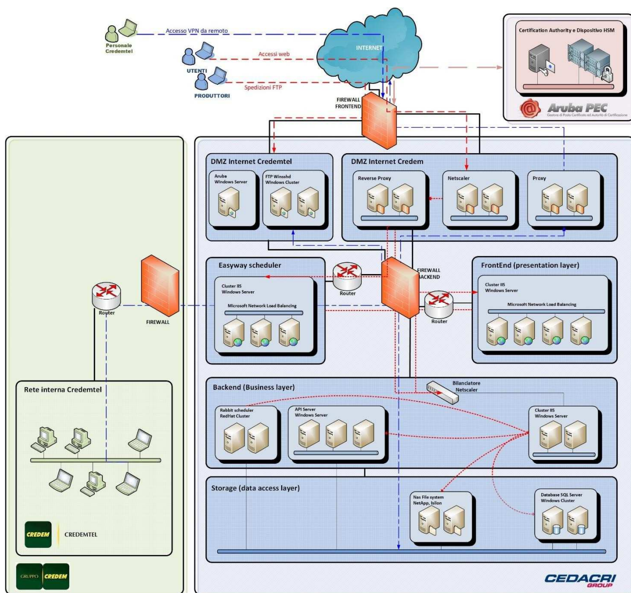
FIGURA 6 COMPONENTI TECNOLOGICHE
