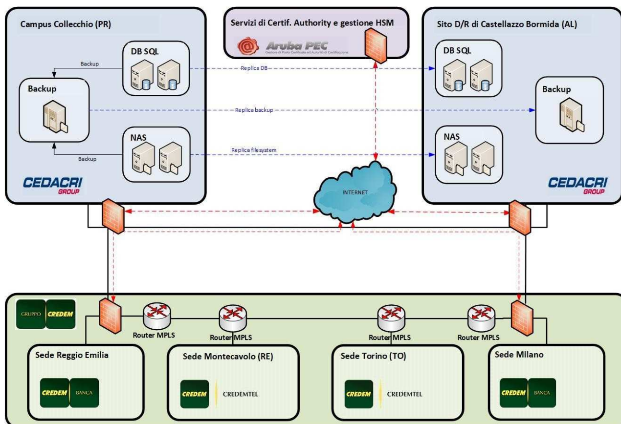
FIGURA 7 COMPONENTI FISICHE
